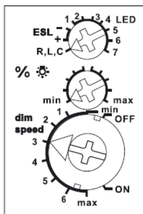
Funksjonsvelgere (Fabrikkinstilling)
